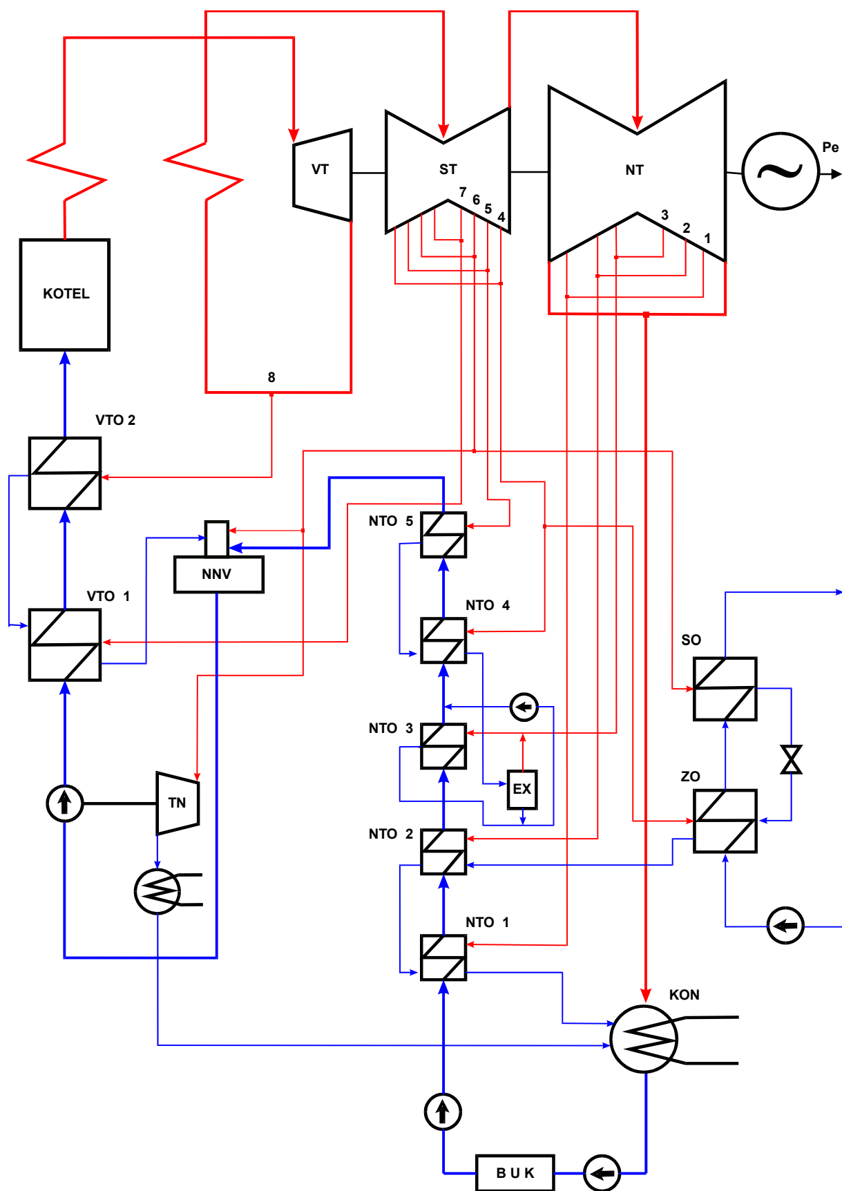
Zjednodušené tepelné schéma tepelného bloku 200 MW v Tušimicích
