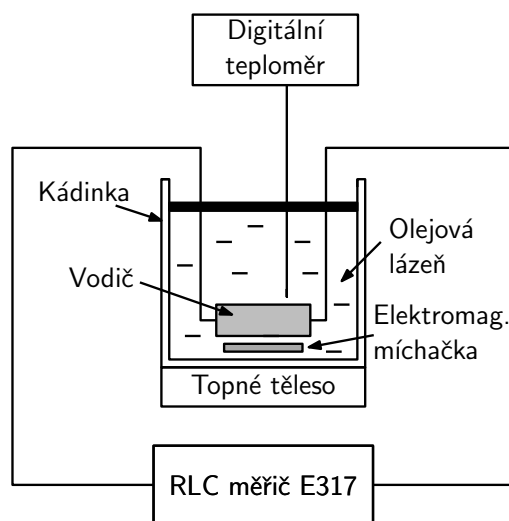
Obr. 1: Schematické znázornění uspořádání experimentu.
