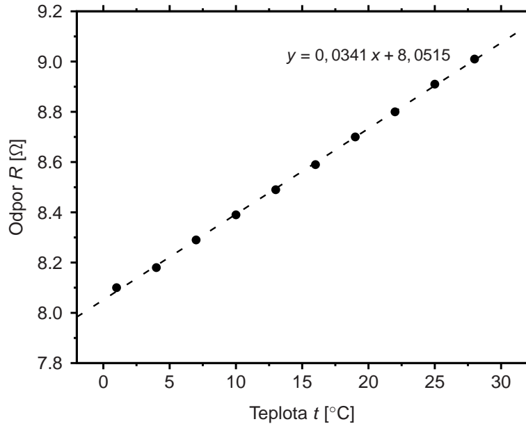
Obr. 2: Naměřená závislost odporu vodiče na teplotě (plné body) a lineární aproximace naměřených hodnot (přerušovaná čára).
