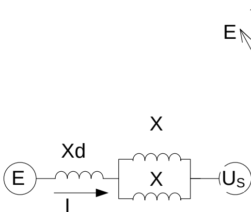
b) náhradní schéma
