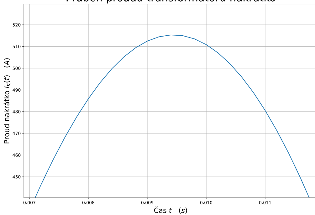
Průběh proudu transformátoru nakrátko
