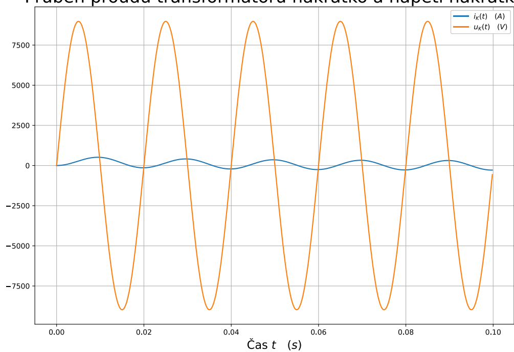
Průběh proudu transformátoru nakrátko a napětí nakrátko
