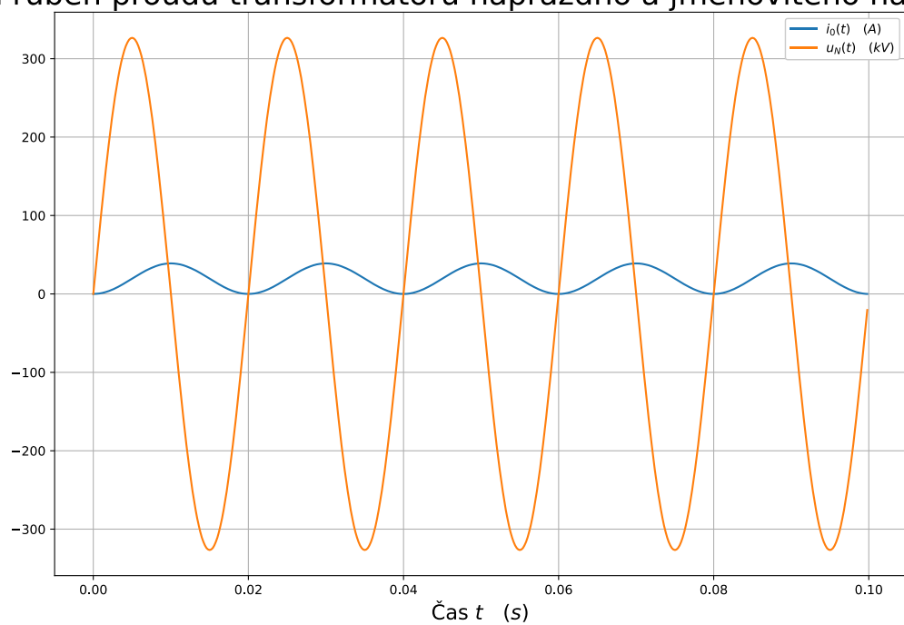
Průběh proudu transformátoru naprázdno a jmenovitého napětí
