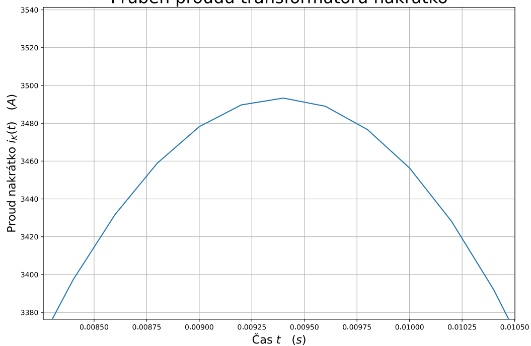
Průběh proudu transformátoru nakrátko
