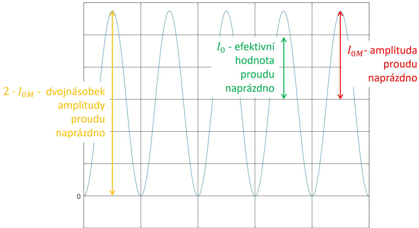
0 Průběh a parametry proudu při zapnutí do stavu naprázdno 0.1
