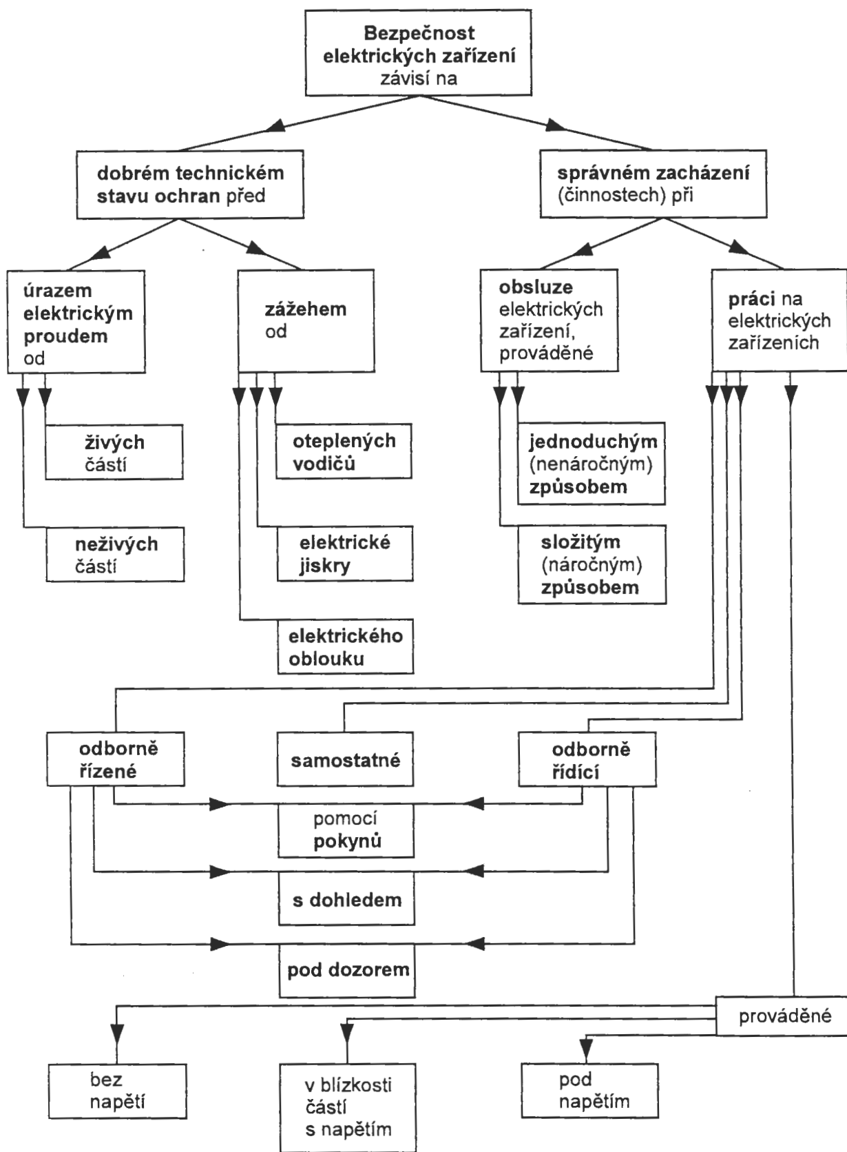
Schéma bezpečnosti elektrických zařízení
