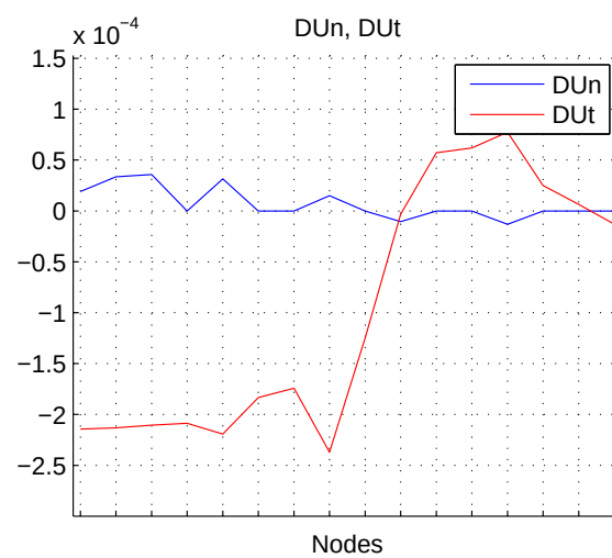
Obrázek 35: Normálová a tečná složka posunutí na kontaktní hranici
