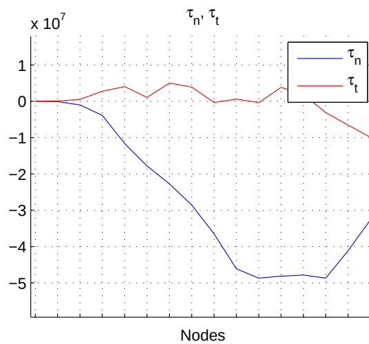
Obrázek 36: Normálová a tečná složka napětí na kontaktní hranici
