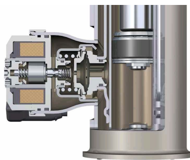
Tlumič CDC (ZF Sachs) – proporcionální ventil uvnitř nebo vně tlumiče
