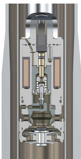
Tlumič CDC (ZF Sachs) – proporcionální ventil uvnitř nebo vně tlumiče
